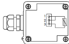
Anschluss bei LM235Z 1=Plus 2=Minus
