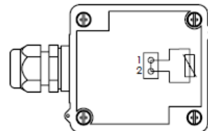
Anschluss bei LM235Z 1=Plus 2=Minus
