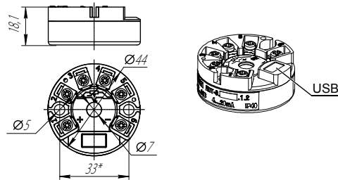
Fig. 1 Dimensions
